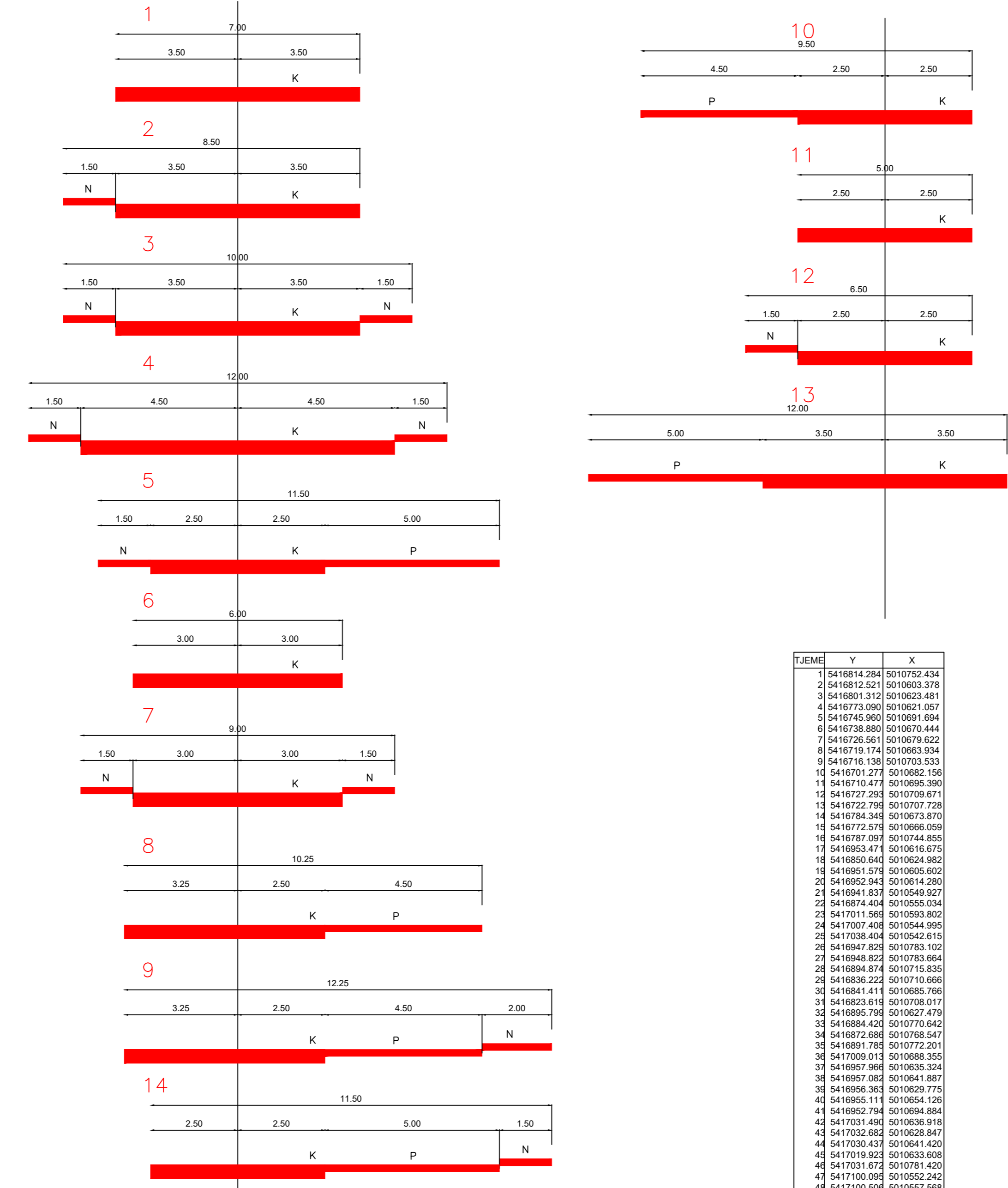
KARAKTERISTIČNI POPREČNI PROFILI M 1:100
