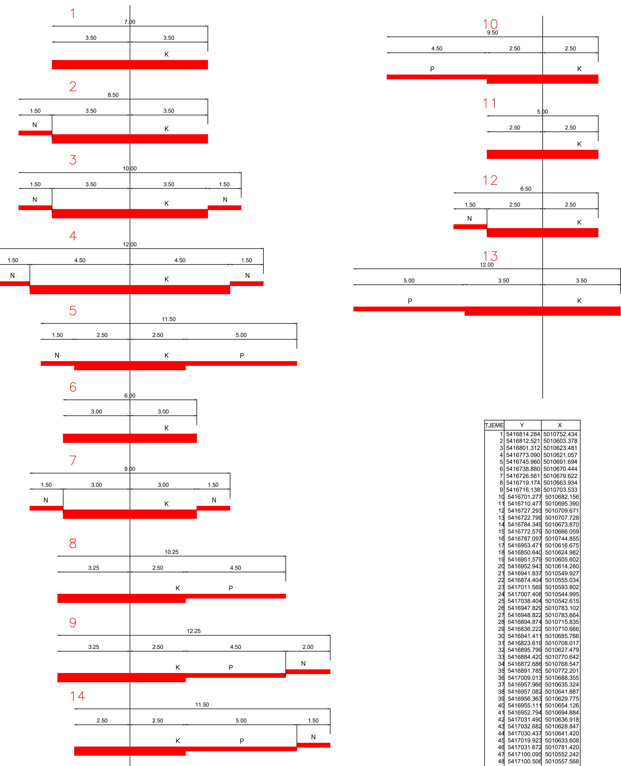
KARAKTERISTIČNI POPREČNI PROFILI M 1:100
